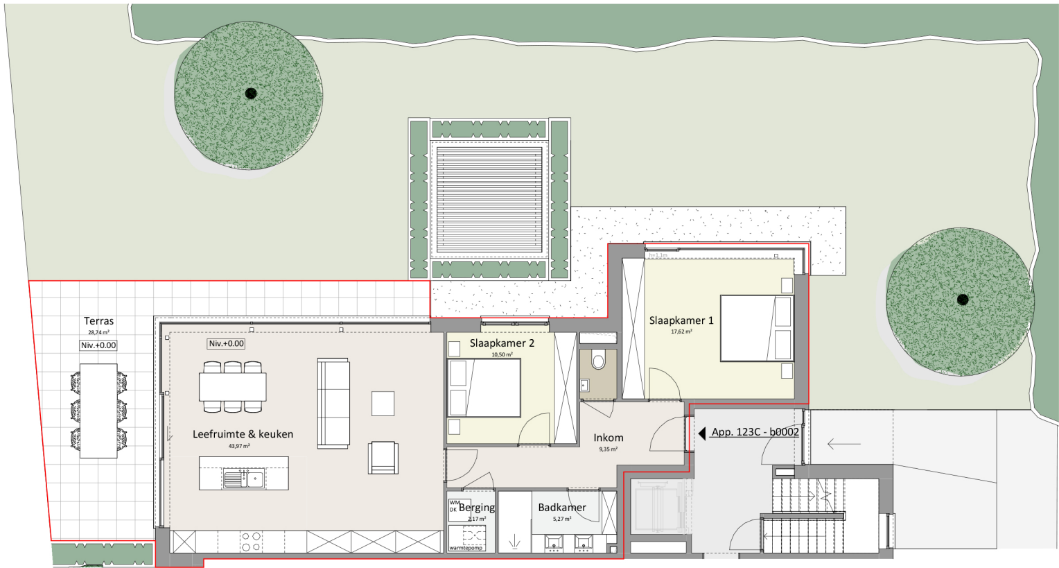
GRONDPLAN - schaal 1/100
